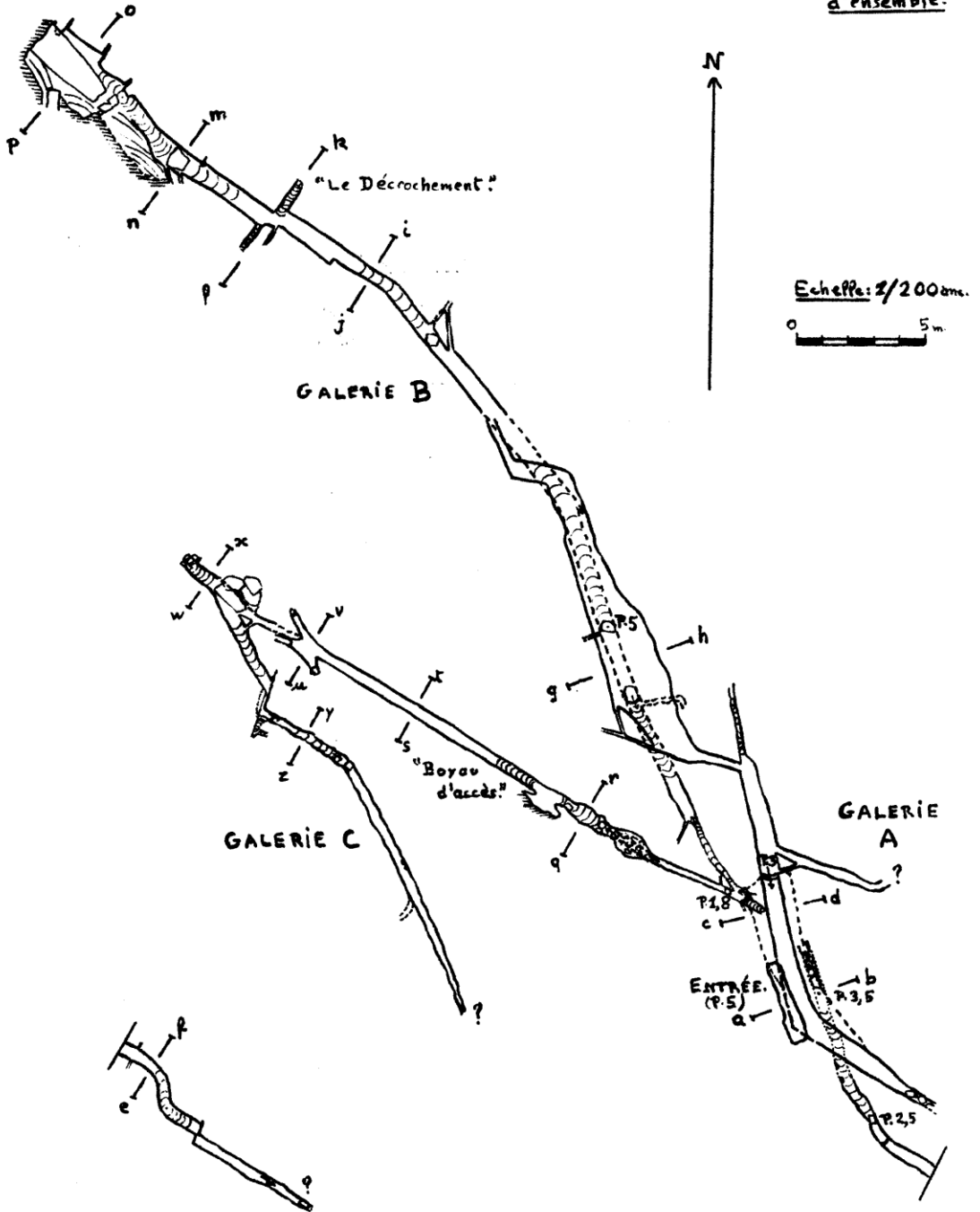
Fig.3 - Plan d'ensemble.
