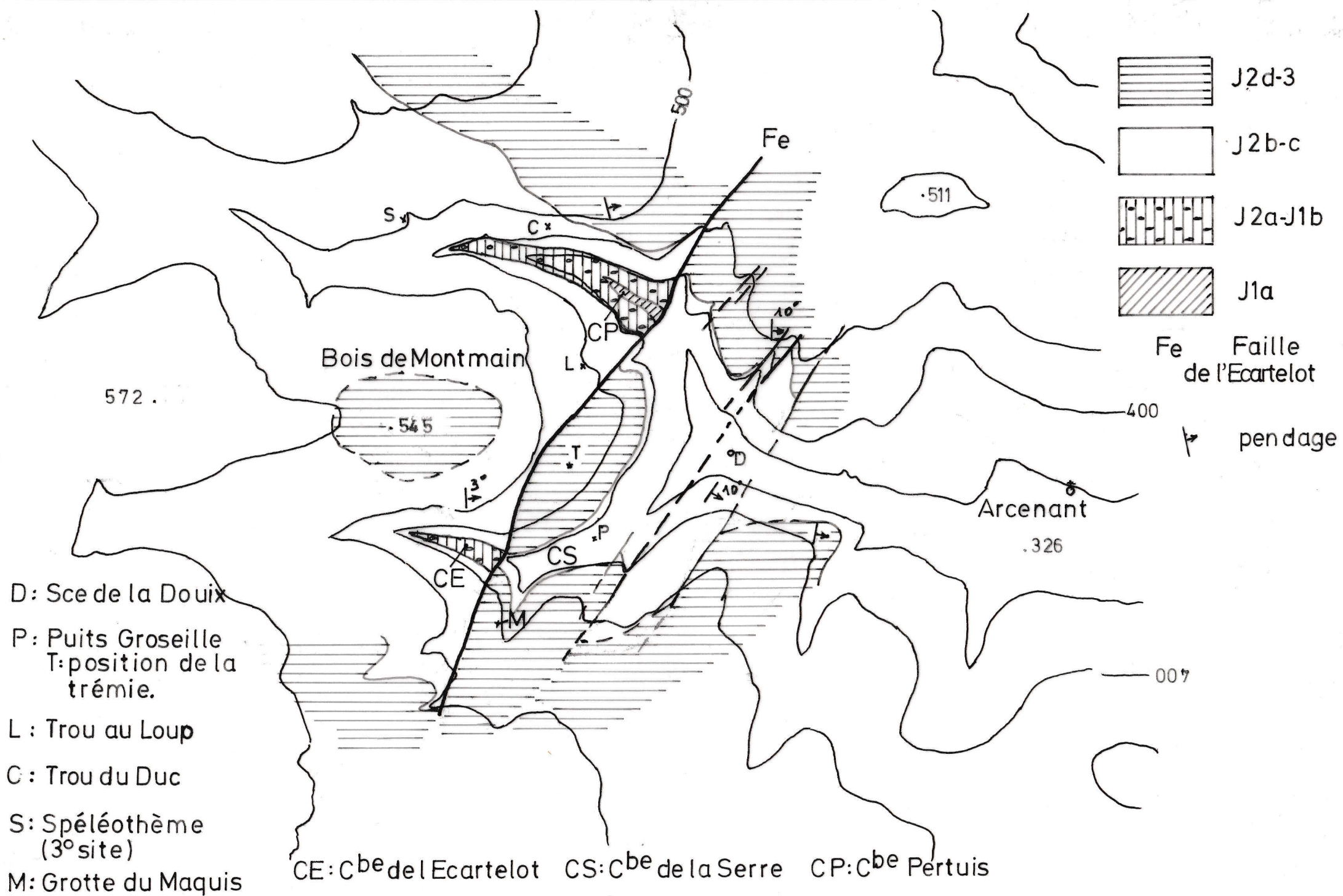
Fig.3-Carte géologique en amont de La Douix
