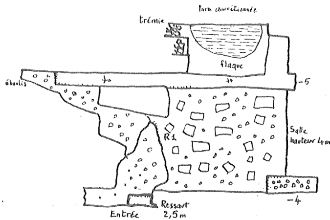
Coupe schématique 1/200°
